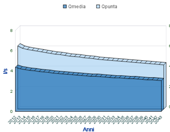
Analisi Portate Comune Di TREVICO
