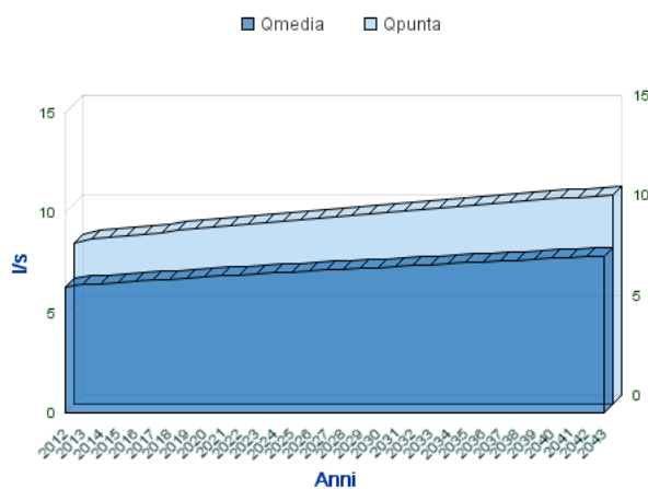
Analisi Portate Comune Di SAN POTITO ULTRA
