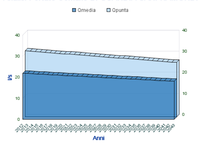
Analisi Portate Comune Di GUARDIA SANFRAMONDI
