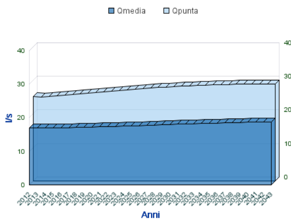
Analisi Portate Comune Di SAN SALVATORE TELESINO
