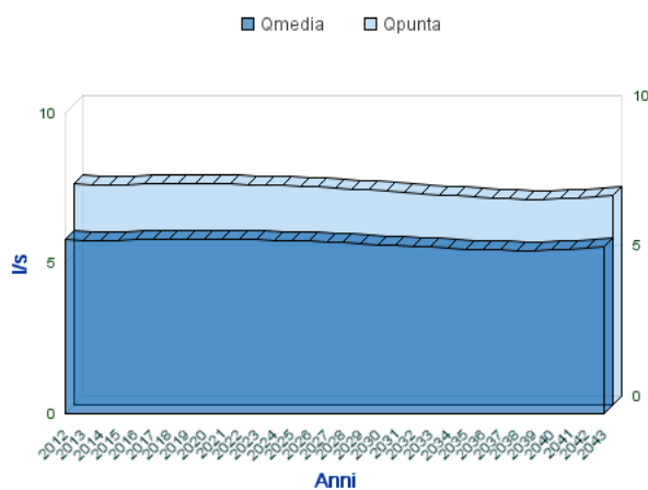
Analisi Portate Comune Di TEORA
