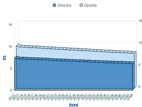
Analisi Portate Comune Di FRAGNETO MONFORTE
