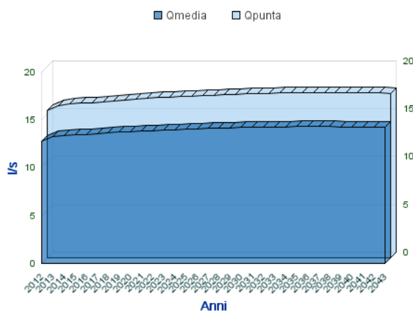
Analisi Portate Comune Di SAN MICHELE DI SERINO
