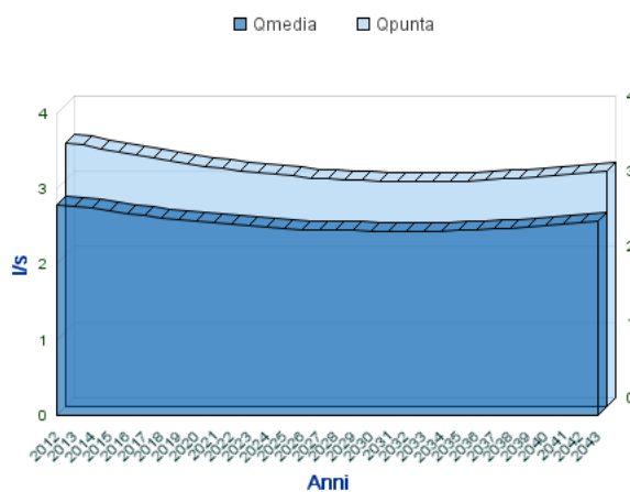
Analisi Portate Comune Di GRECI
