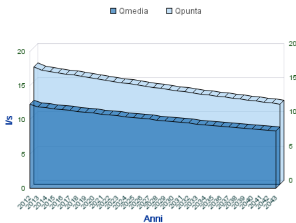
Analisi Portate Comune Di VALLATA
