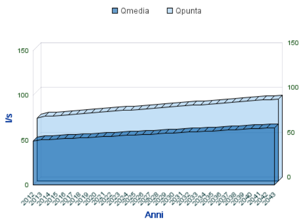
Analisi Portate Comune Di MONTORO INFERIORE
