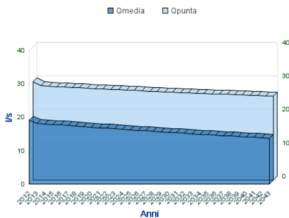
Analisi Portate Comune Di PADULI
