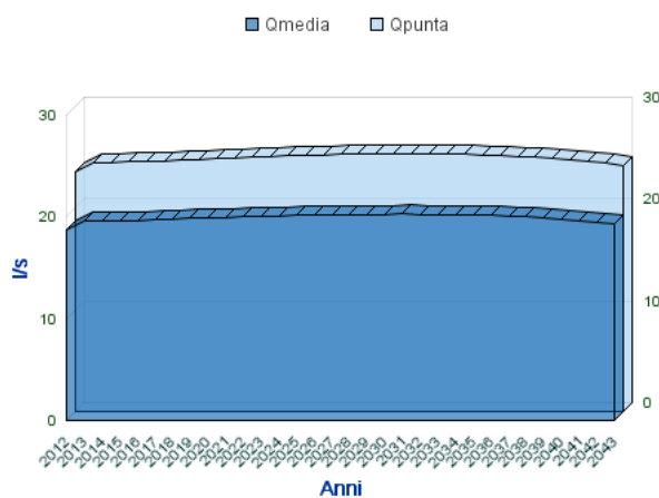
Analisi Portate Comune Di SANT'ANGELO DEI LOMBARDI
