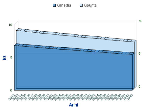
Analisi Portate Comune Di LAPIO
