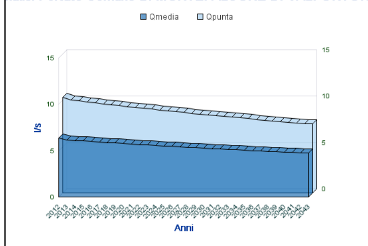
Analisi Portate Comune Di MONTEFALCONE DI VALFORTORE
