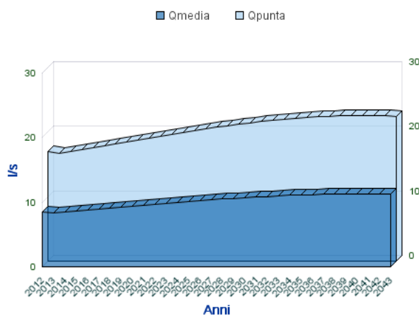
Analisi Portate Comune Di OSPEDALETTO D'ALPINOLO
