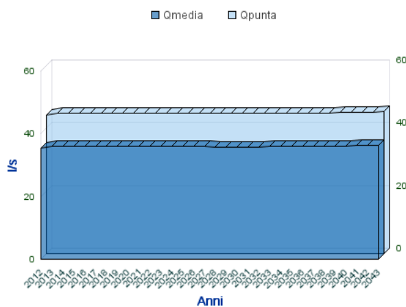
Analisi Portate Comune Di SERINO
