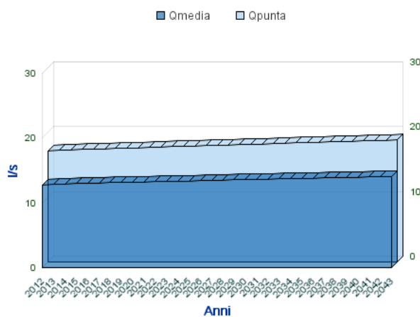
Analisi Portate Comune Di PONTE
