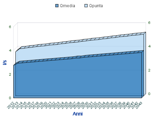
Analisi Portate Comune Di SANT'ANGELO A SCALA
