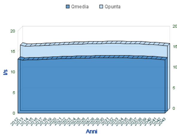
Analisi Portate Comune Di PRATA DI PRINCIPATO ULTRA
