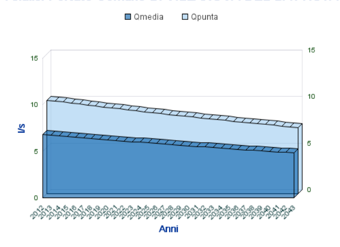
Analisi Portate Comune Di VILLANOVA DEL BATTISTA
