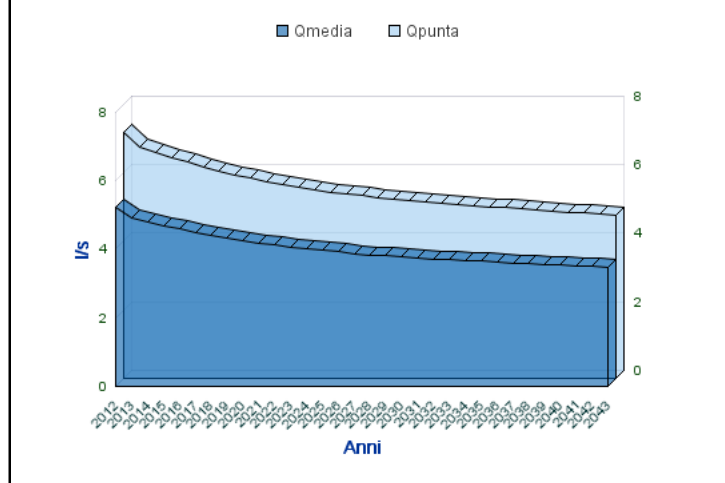
Analisi Portate Comune Di CASTELVETERE IN VALFORTORE
