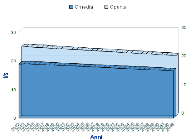
Analisi Portate Comune Di SAN MARCO DEI CAVOTI
