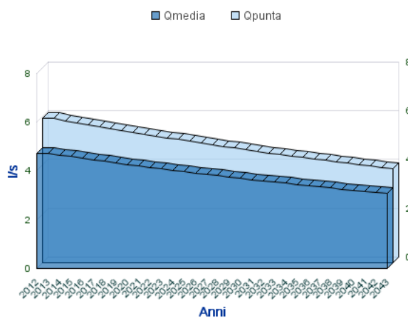
Analisi Portate Comune Di ZUNGOLI
