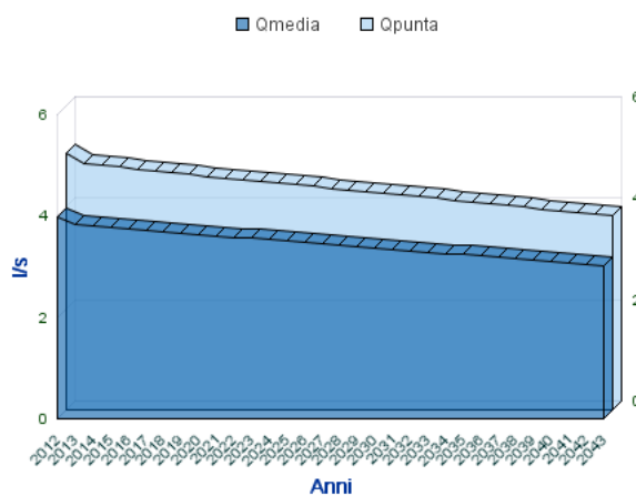
Analisi Portate Comune Di TUFO
