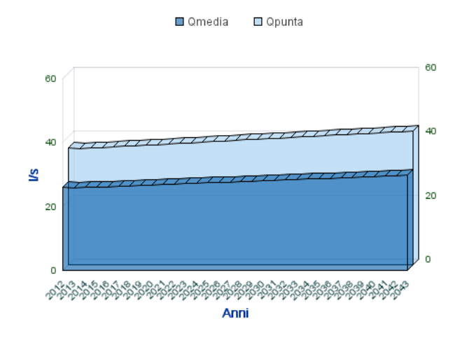
Analisi Portate Comune Di MUGNANO DEL CARDINALE
