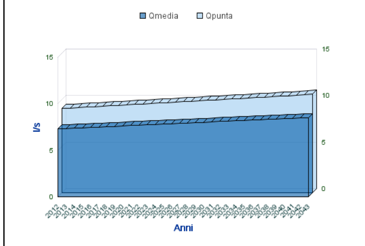
Analisi Portate Comune Di PAGO DEL VALLO DI LAURO
