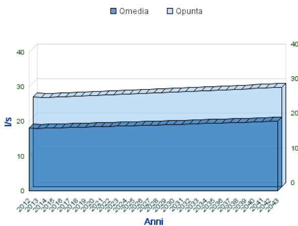
Analisi Portate Comune Di S. ANGELO A CUPOLO
