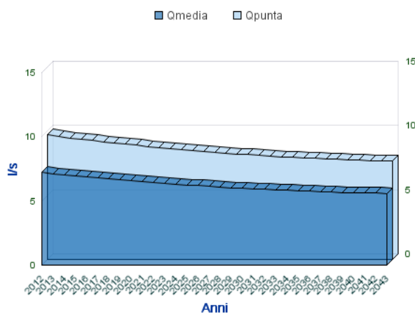
Analisi Portate Comune Di GUARDIA LOMBARDI
