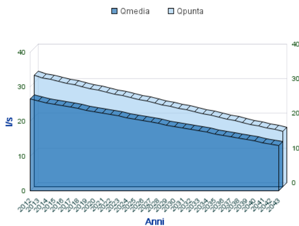
Analisi Portate Comune Di CALITRI
