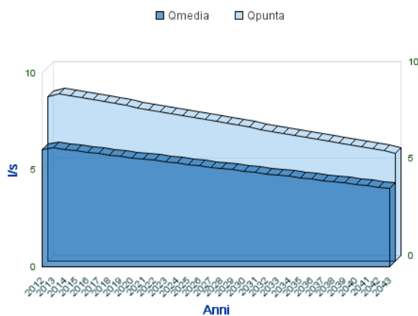
Analisi Portate Comune Di SANT'ANDREA DI CONZA
