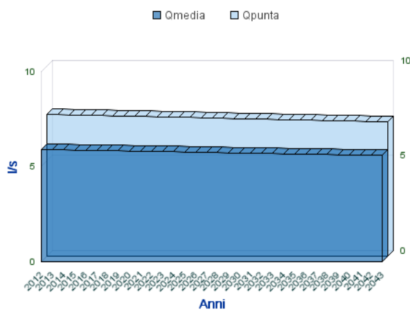
Analisi Portate Comune Di CONZA DELLA CAMPANIA
