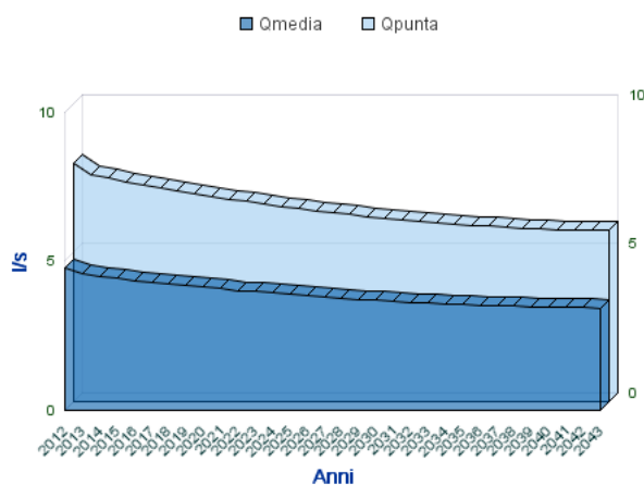
Analisi Portate Comune Di SAVIGNANO IRPINO
