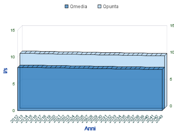
Analisi Portate Comune Di S. LORENZO MAGGIORE
