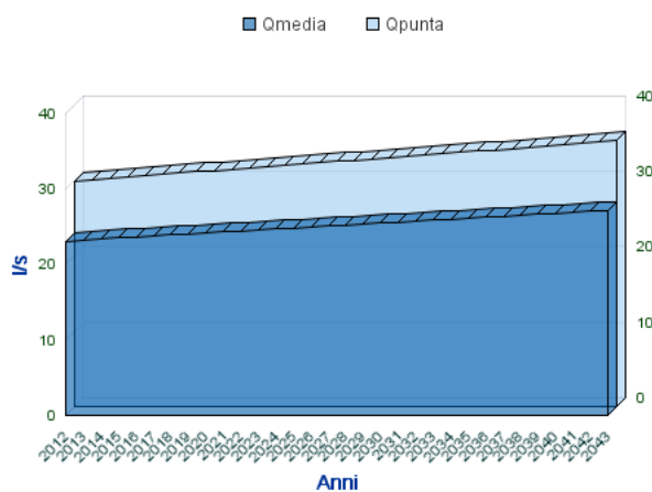
Analisi Portate Comune Di FORINO
