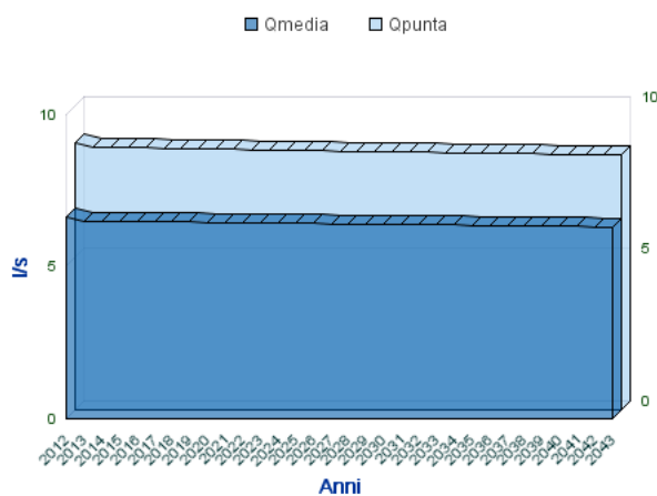
Analisi Portate Comune Di CAMPOLI DEL MONTE TABURNO
