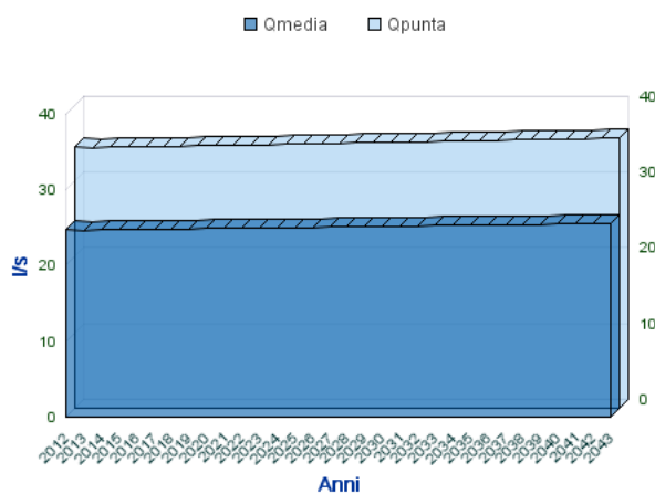
Analisi Portate Comune Di APICE
