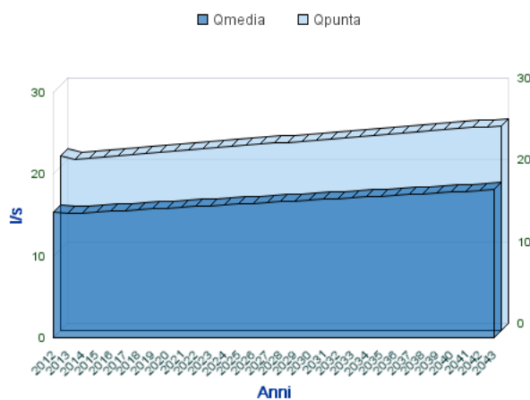
Analisi Portate Comune Di SAN NICOLA MANFREDI
