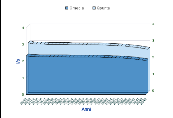
Analisi Portate Comune Di SANT'ARCANGELO TRIMONTE
