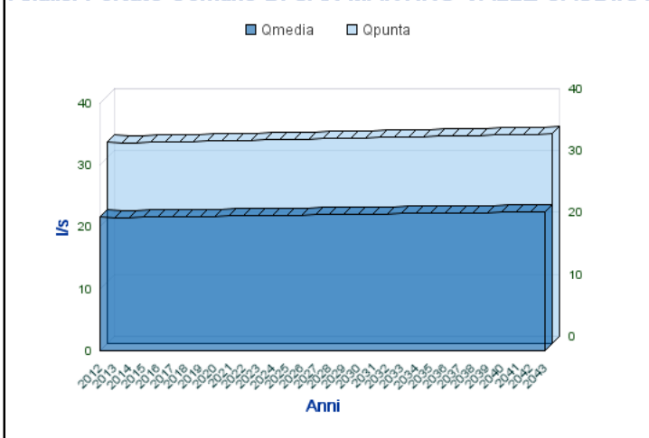
Analisi Portate Comune Di SAN MARTINO VALLE CAUDINA
