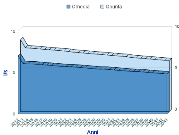
Analisi Portate Comune Di MORRA DE SANCTIS
