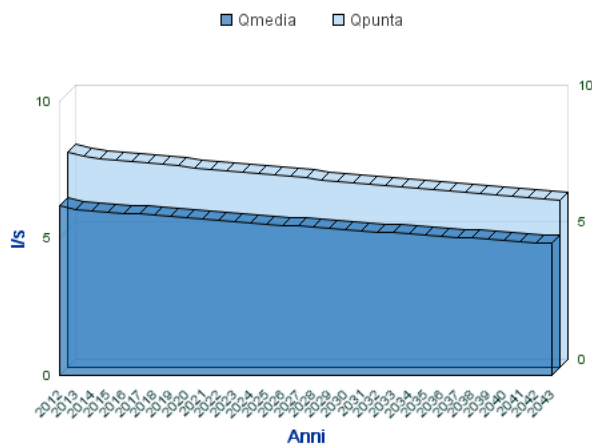
Analisi Portate Comune Di FOIANO IN VALFORTORE
